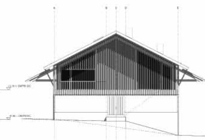
Ansicht Nord
